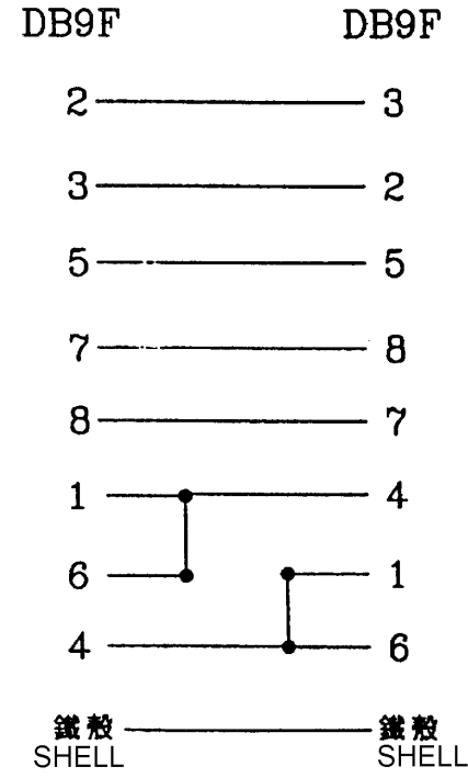
接線表
