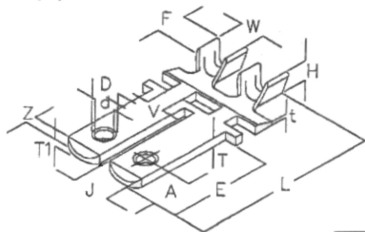
FIG : 插頭片
