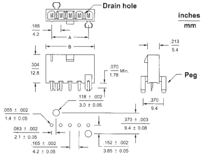
P.C.B. hole dimensions
