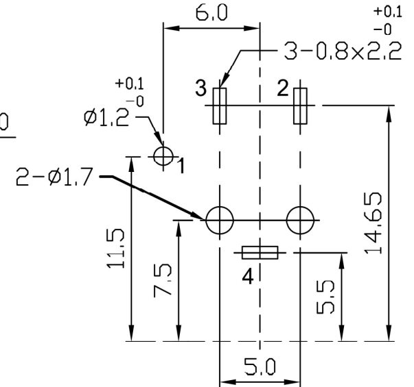
P.C.B LAYOUT(±0.1) (BOTTOM VIEW)
